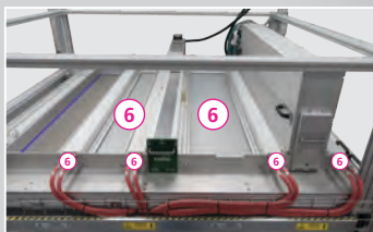
Vue aérienne - Chambre inerte avec injecteurs d'azote réglables
